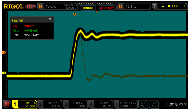
Figura 2.6: La función de prueba paso/fallo puede realizar rápidamente estadísticas sobre la probabilidad de ocurrencia de las excepciones de señal.
